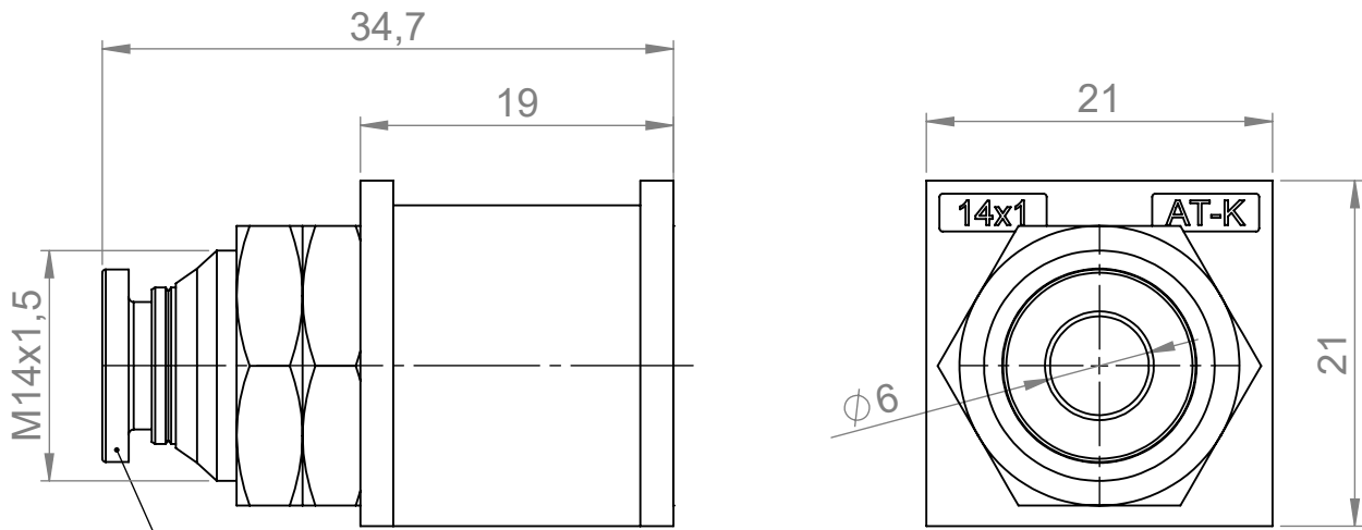
Schottkupplung für Pneumatikschlauch Ø6mm (Bulkhead coupling for pneumatic pipe Ø6mm)
